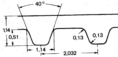
Type MXL (nur Mittelwerte/nominal dimensions - mm)
