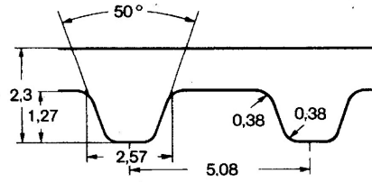
Type XL (nur Mittelwerte/nominal dimensions – mm)
